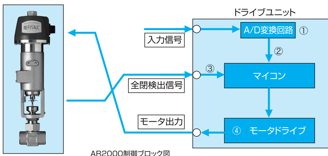
AR2000制御ブロック図
