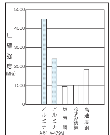
圧縮強度比較図
