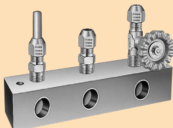
取付例
