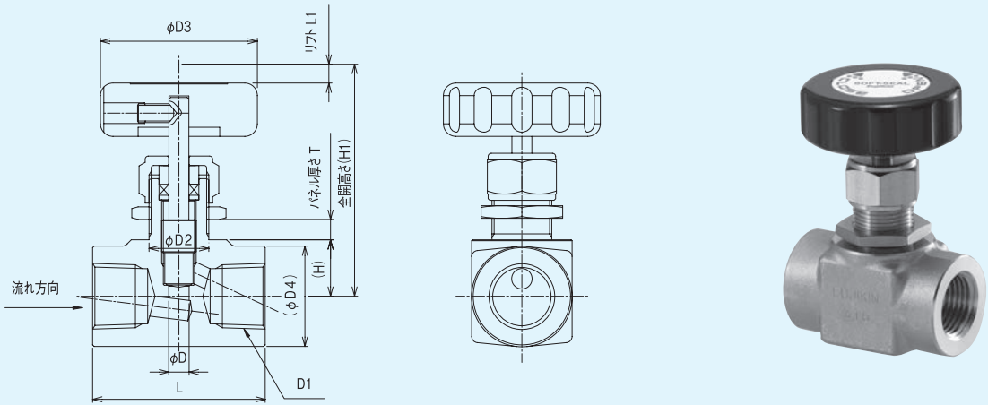
●寸法表
