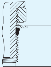
図2 継手の仮締め
