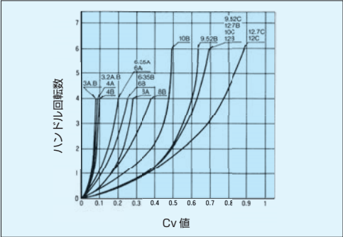
●Cv値曲線
