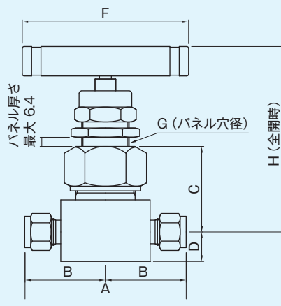
VUH-968 シリーズ
