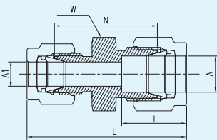
熱電対用対応品
