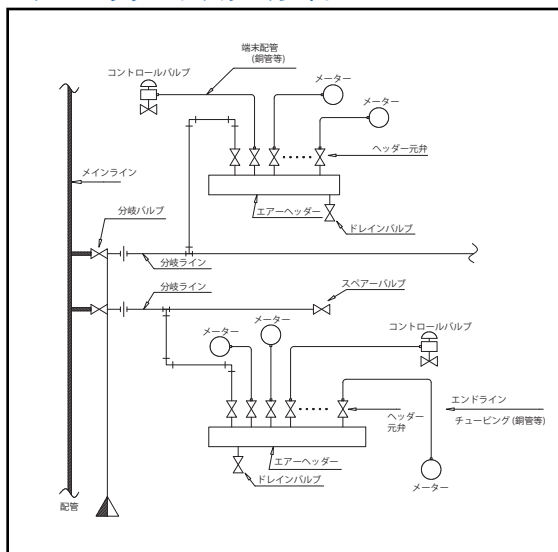
エアヘッダーシステムライン
