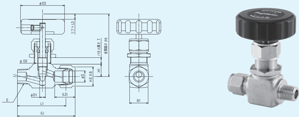
●寸法表(ミリサイズ)
