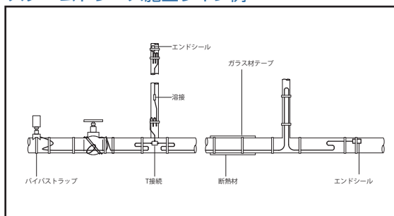
ガスサンプリングライン
