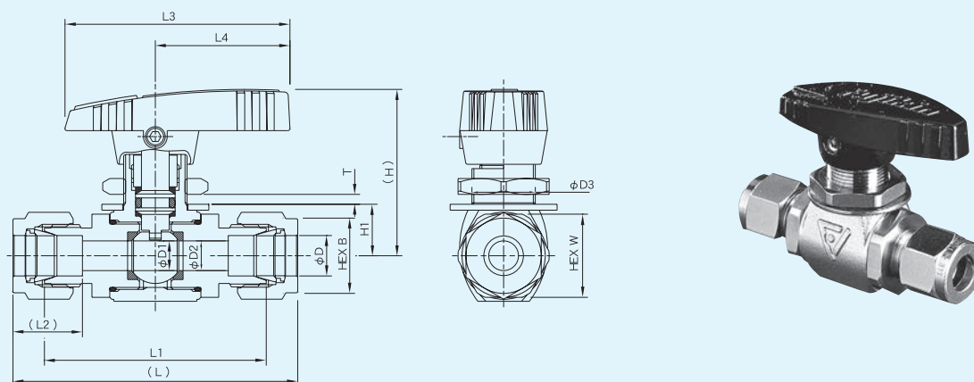
●寸法表(ミリサイズ)
