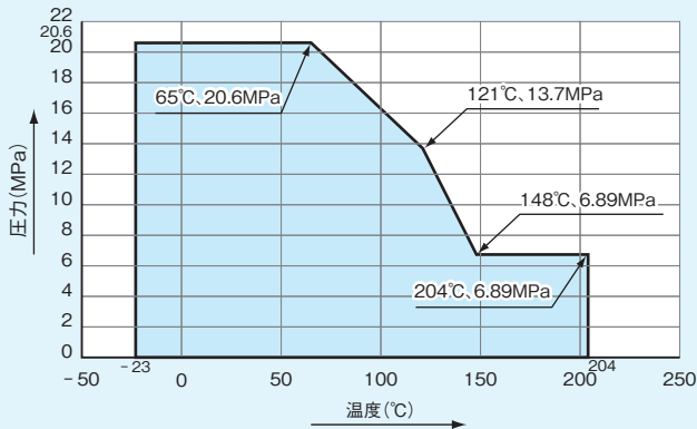
温度・圧力線図
